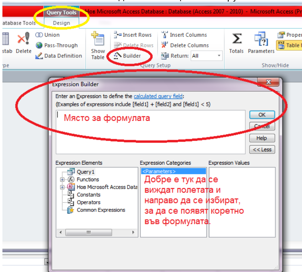
Фиг. 3.1 Място и начин за създаване на формула за изчисление
