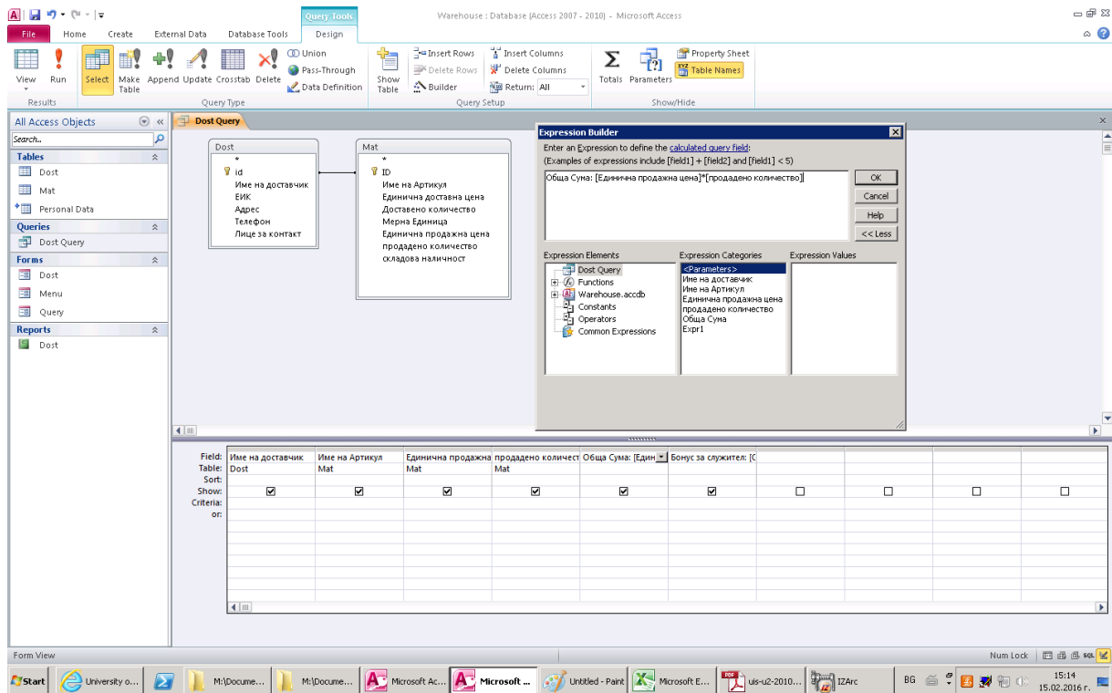
Фиг. 3.2 Пример за изчисление на „Обща сума“
