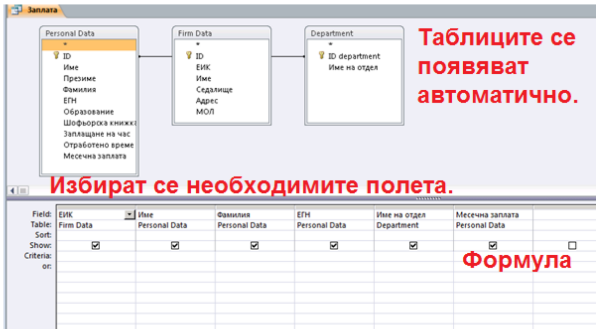
Фиг. 3. Примерен изглед от режим Query Design
